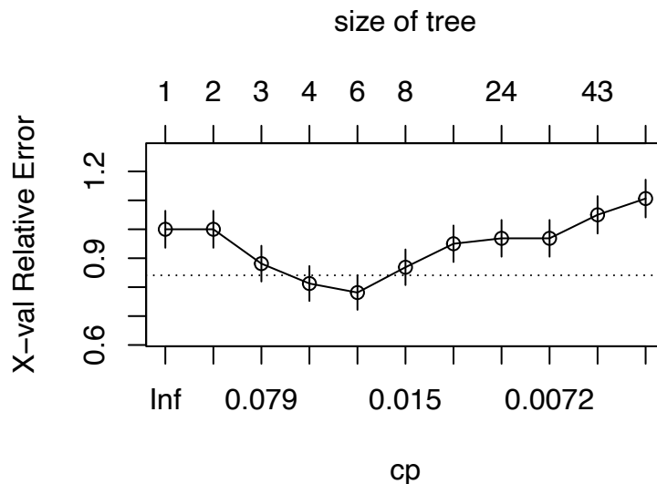
Figure 8.14 – Erreur de prévision en fonction de la complexité.
