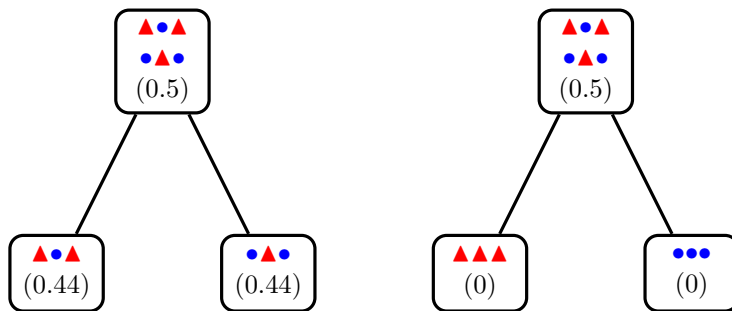
Figure 8.7 – 2 exemples de coupure d'un même nœud, l'impureté de Gini est précisée entre parenthèses).
