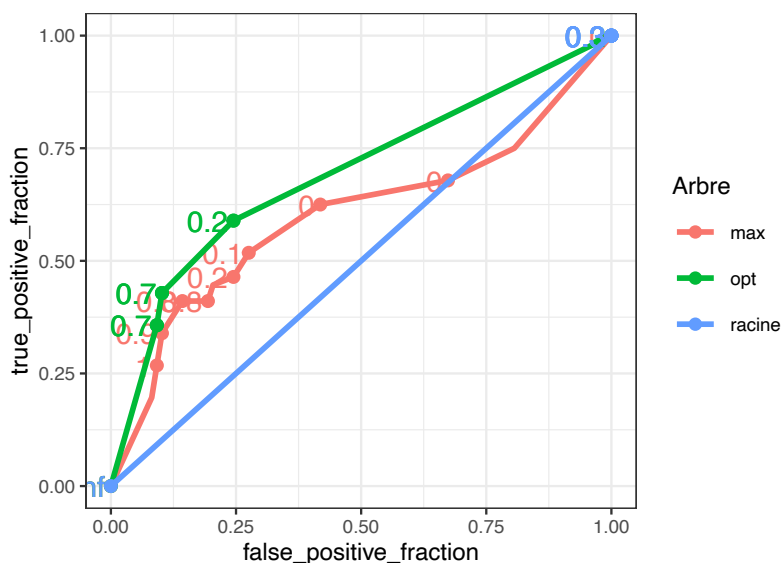
Figure 8.20 – Comparaison des courbes ROC par hold out.
