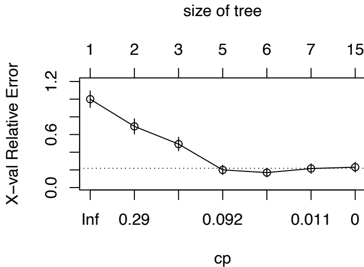
Figure 8.11 – Choix de la complexité de l'arbre avec 'plotcp'.
