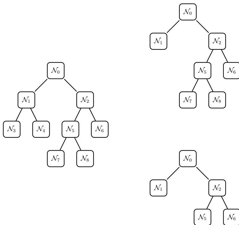
Figure 8.8 – 2 sous-arbres (droite) d'un même arbre (gauche).
