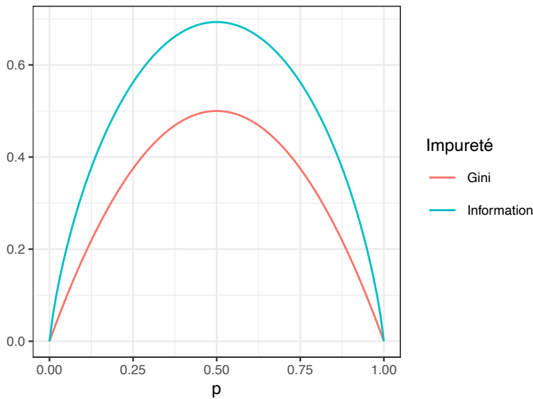
Figure 8.6 – Impuretés de Gini et d'information.
