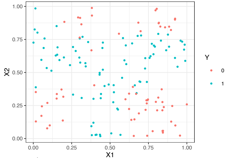
Figure 8.1 – Échantillon de taille 150 avec 2 variables explicatives et une variable binaire à expliquer.
