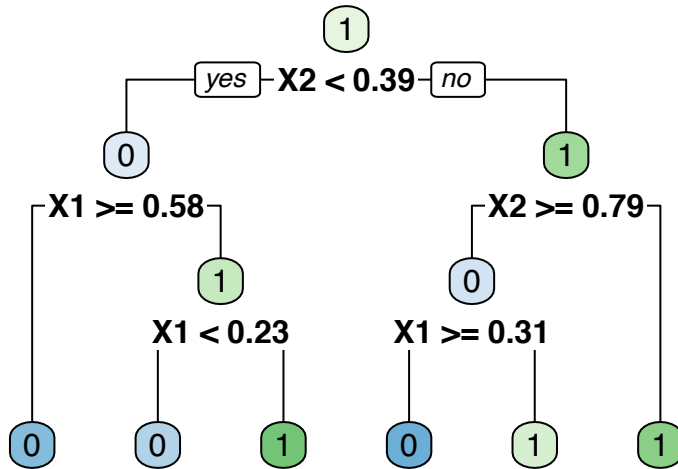
Figure 8.3 – Arbre correspondant à la figure 8.2.
