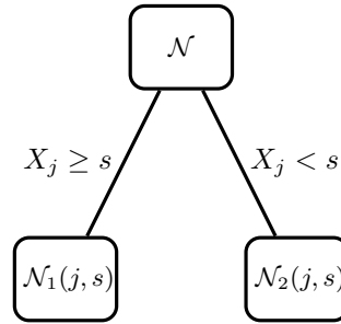
Figure 8.4 – \mathcal{N} et ses 2 nœuds fils.
