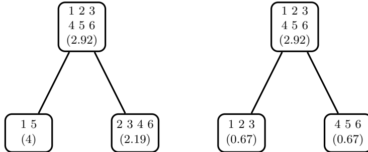
Figure 8.5 – 2 exemples de coupure d'un même nœud, l'impureté est précisée entre parenthèses.
