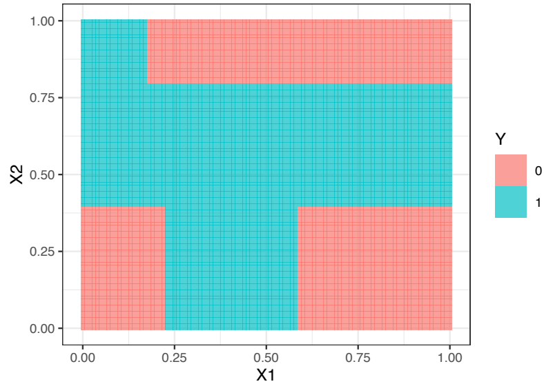
Figure 8.13 – Les prévisions de l’arbre optimal.
