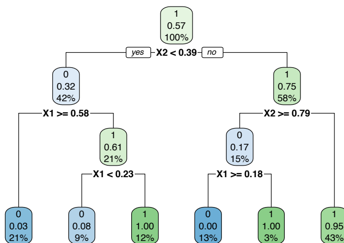
Figure 8.12 – Représentation de l'arbre optimal
