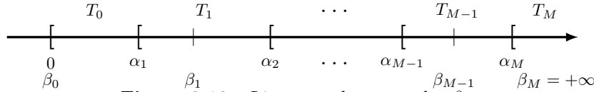
Figure 8.10 – Lien entre les \alpha_m et les \beta_m .
